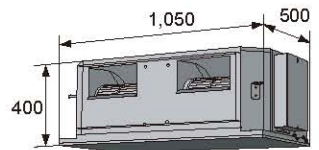
ARXC36LATH : 45kg (unit: mm)
